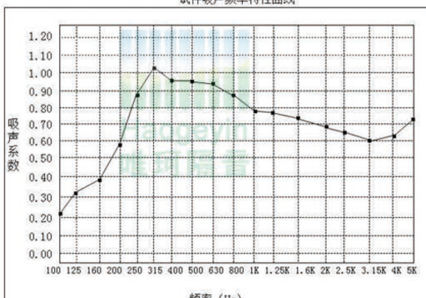
试件吸声频率特性曲线
